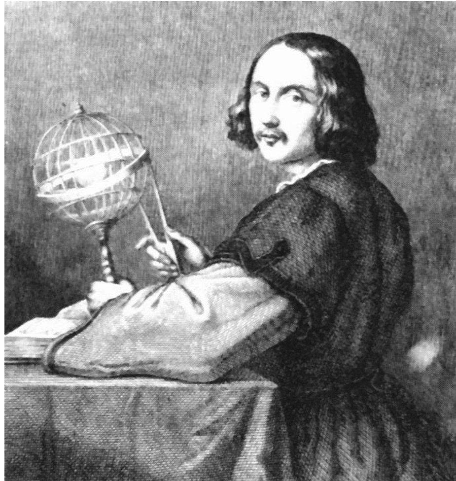
Copernicus
